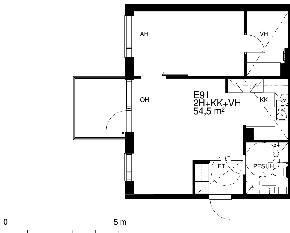
Pohjapiirros 1:100
