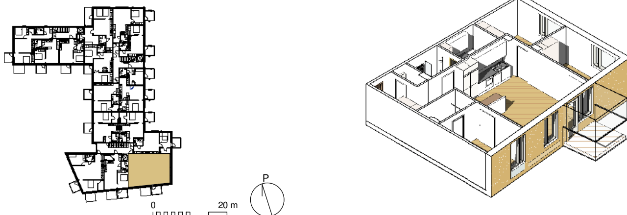
Sijainti 1:1000
