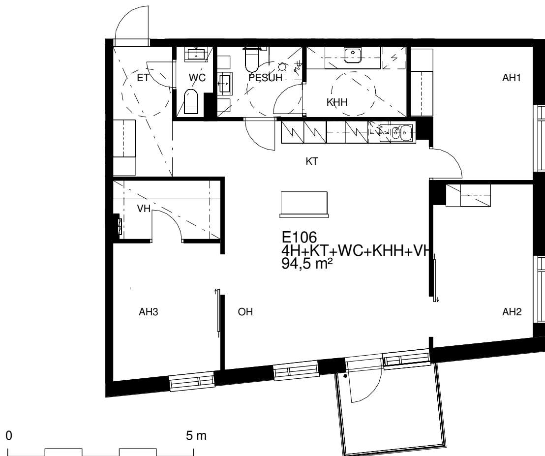
Pohjapiirros 1:100
