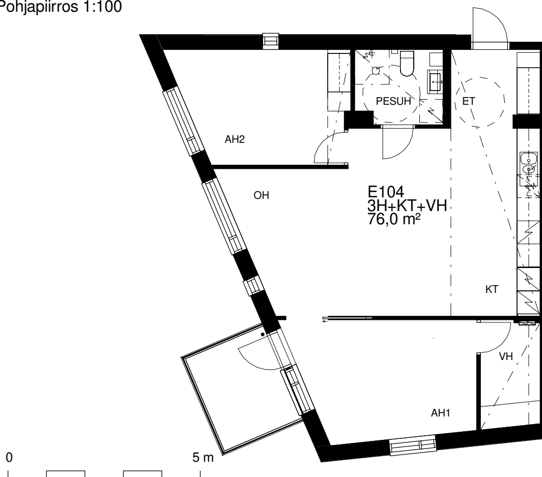
Pohjapiirros 1:100
