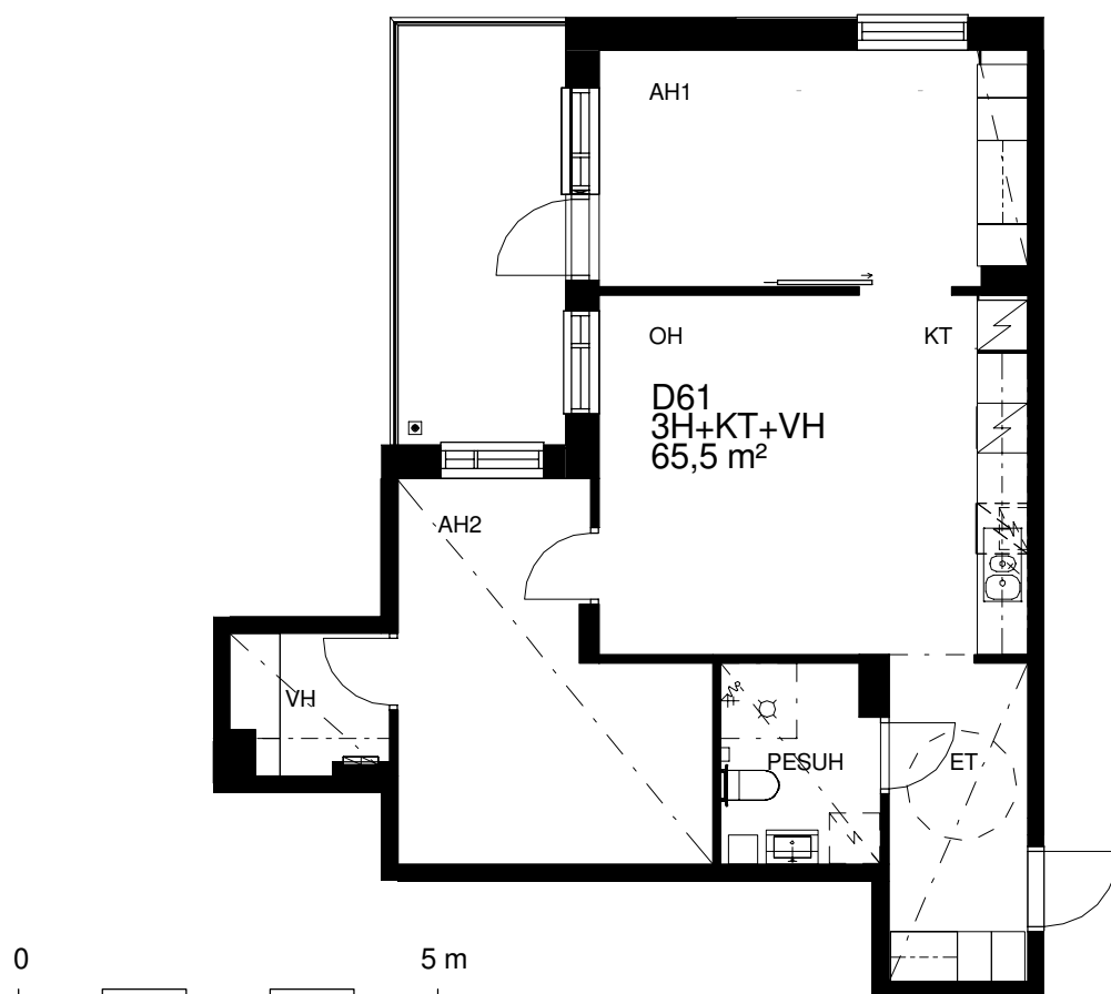
Pohjapiirros 1:100
