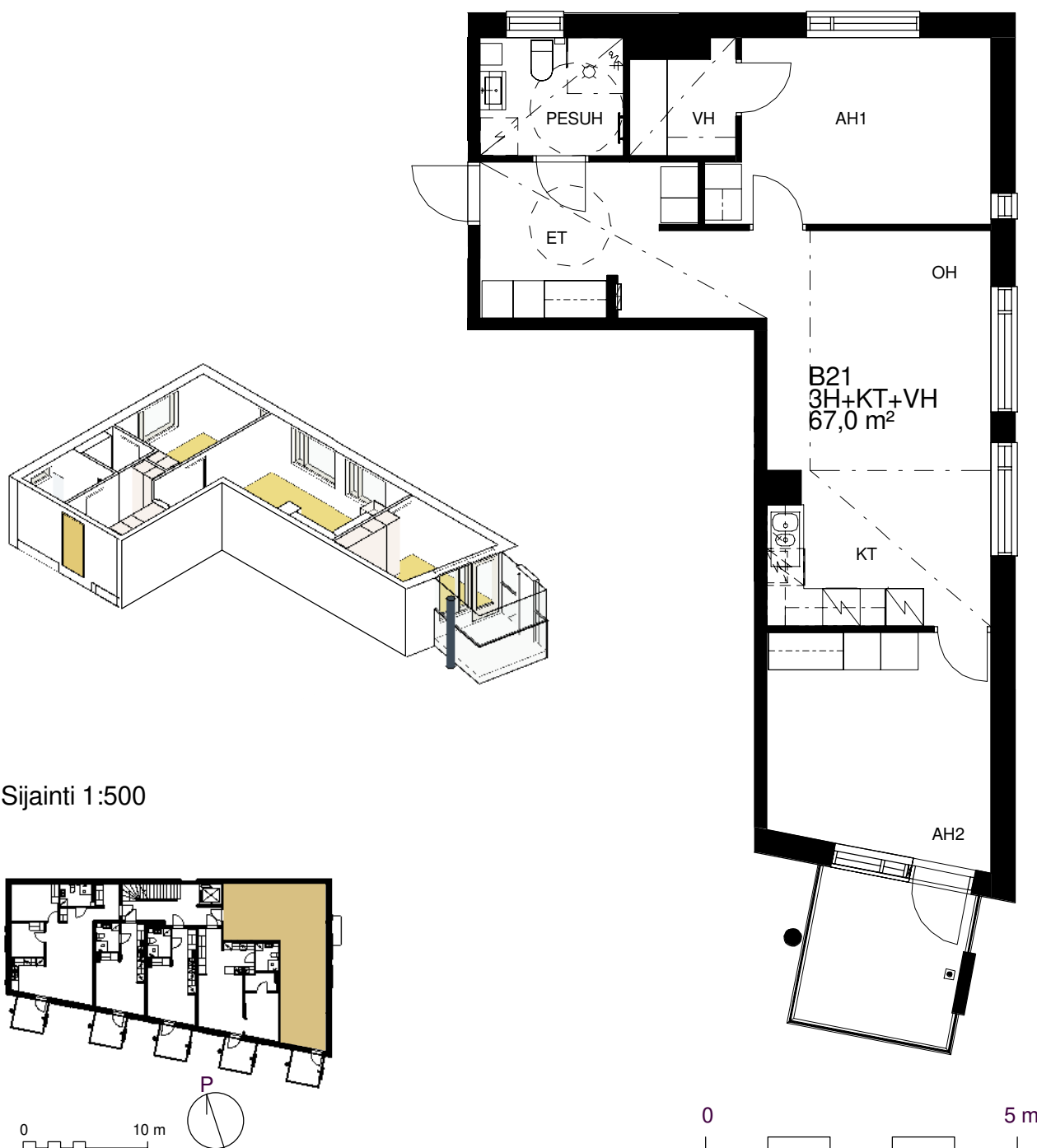
Pohjapiirros 1:100
