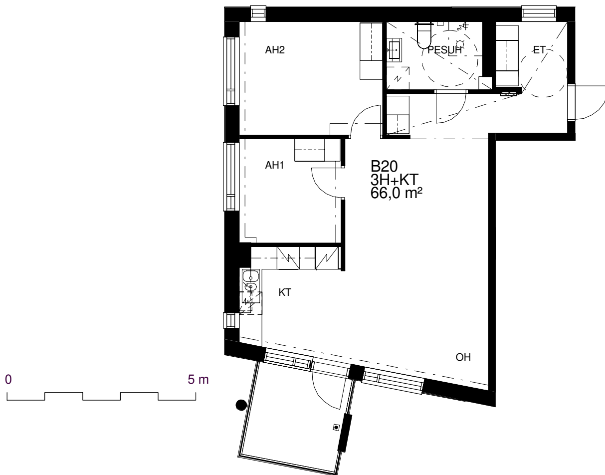
Pohjapiirros 1:100
