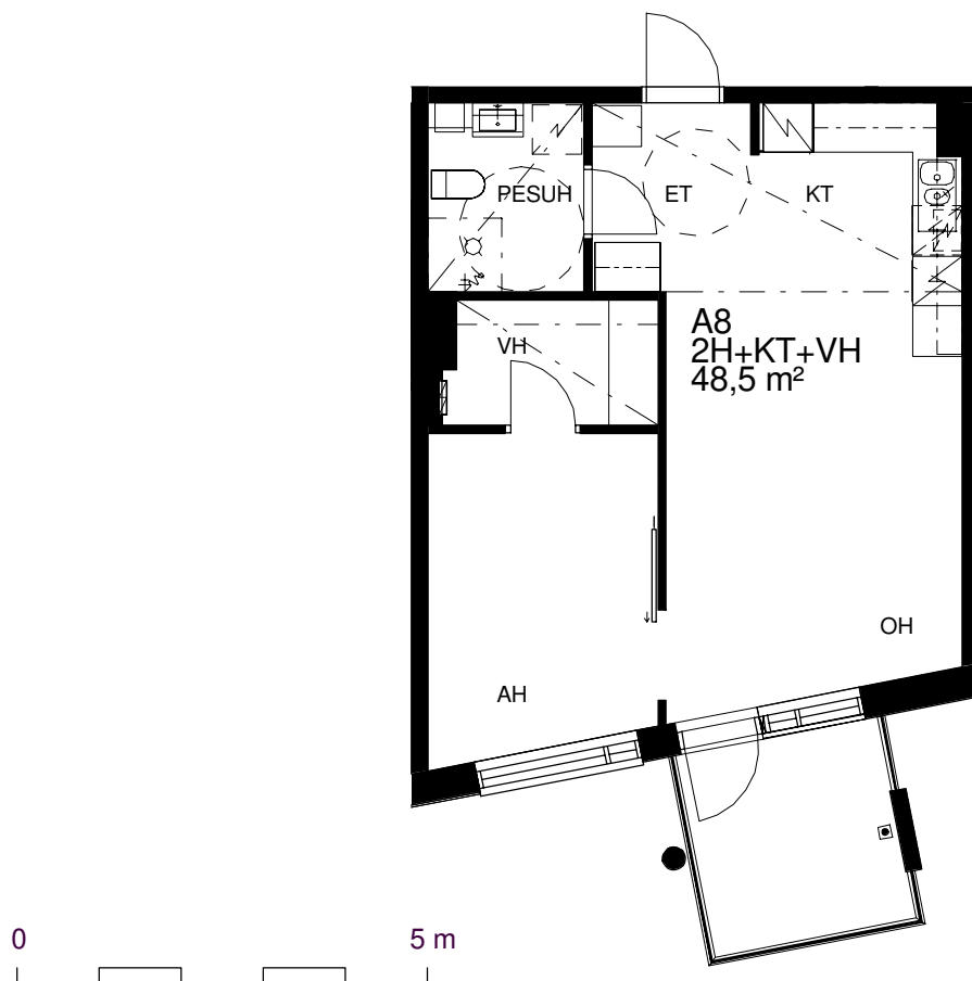
Pohjapiirros 1:100
