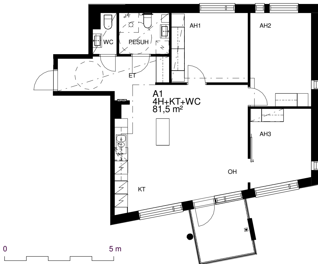
Pohjapiirros 1:100
