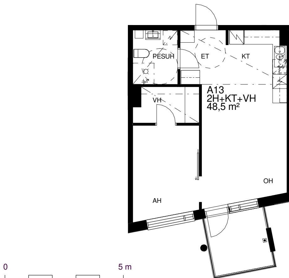
Pohjapiirros 1:100
