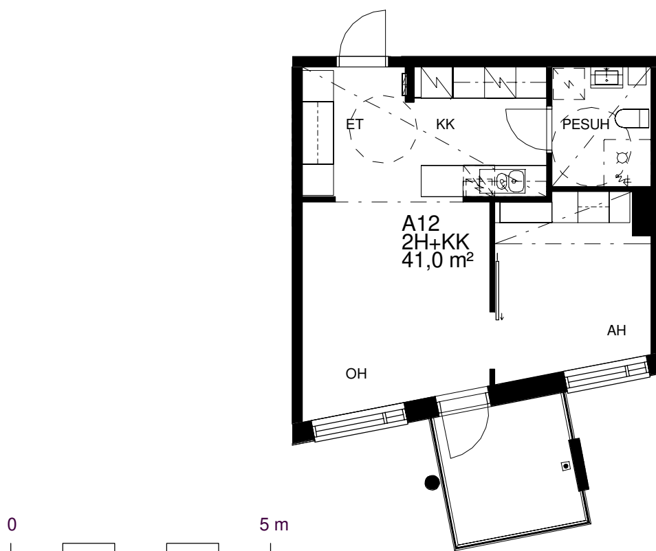
Pohjapiirros 1:100
