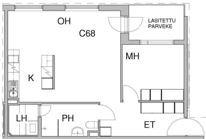
Pohjapiirros, 1:100
