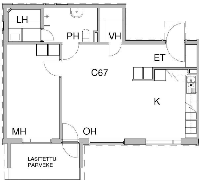
Pohjapiirros, 1:100
