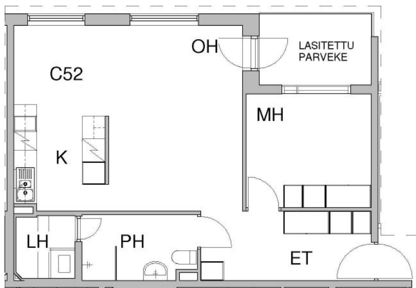
Pohjapiirros, 1:100
