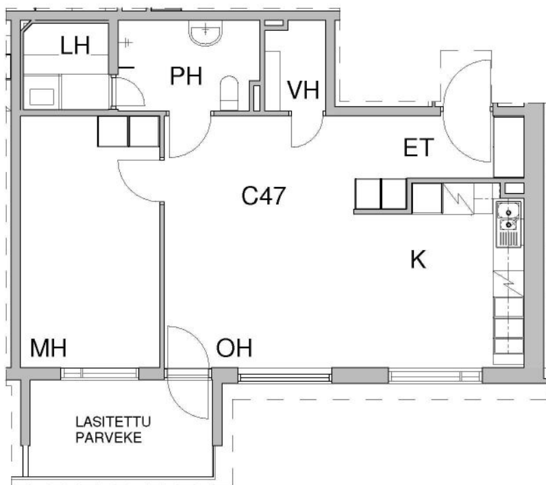
Pohjapiirros, 1:100
