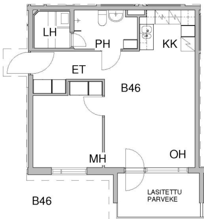
Pohjapiirros, 1:100
