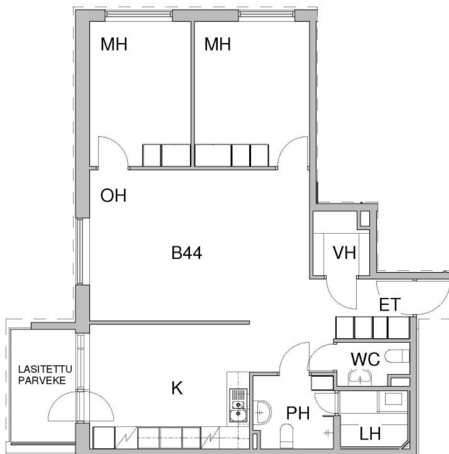
Pohjapiirros, 1:100
