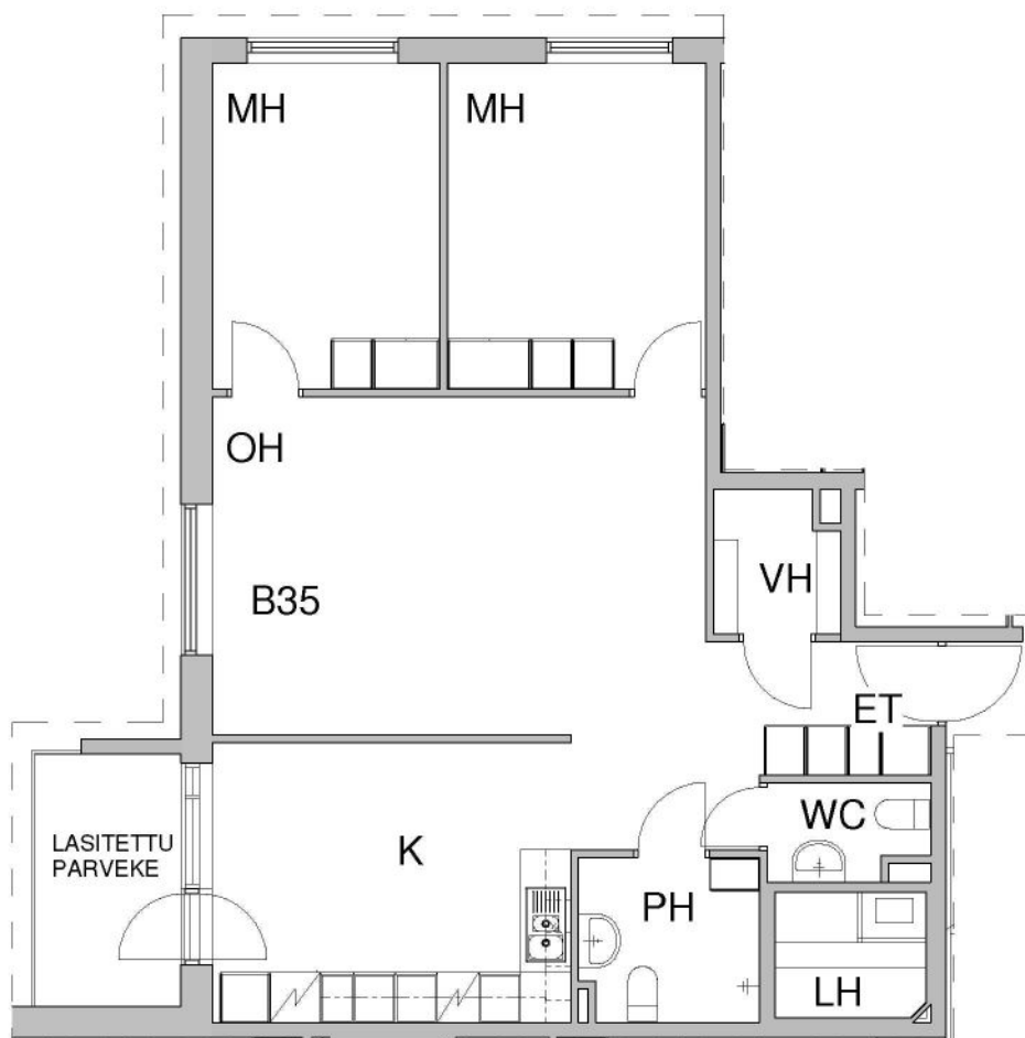
Pohjapiirros, 1:100
