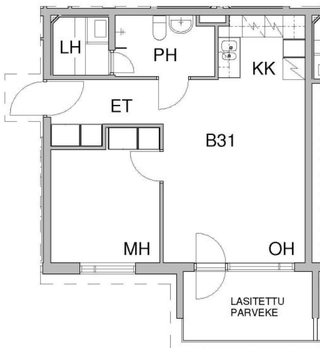
Pohjapiirros, 1:100
