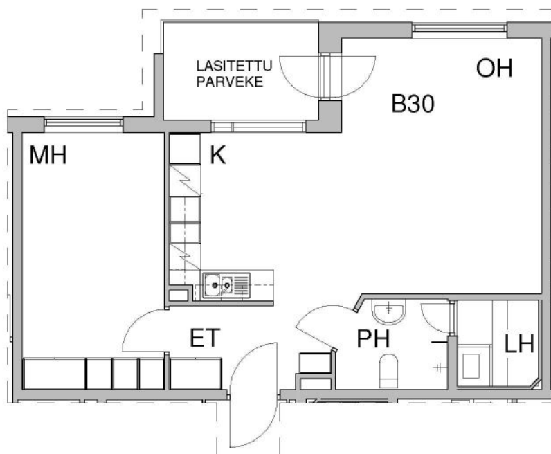
Pohjapiirros, 1:100
