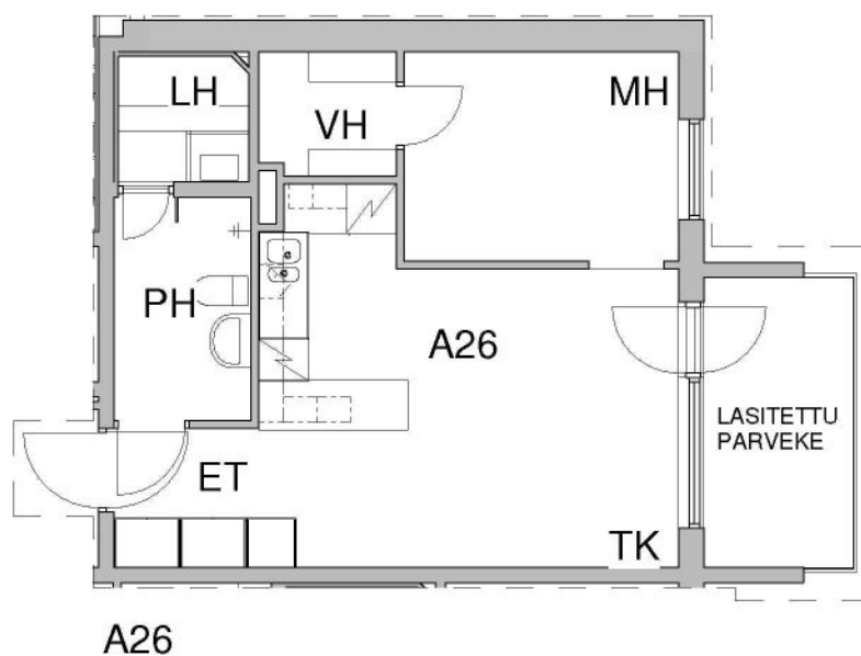
Pohjapiirros, 1:100
