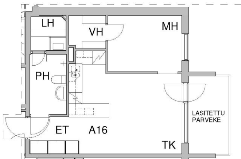
Pohjapiirros, 1:100
