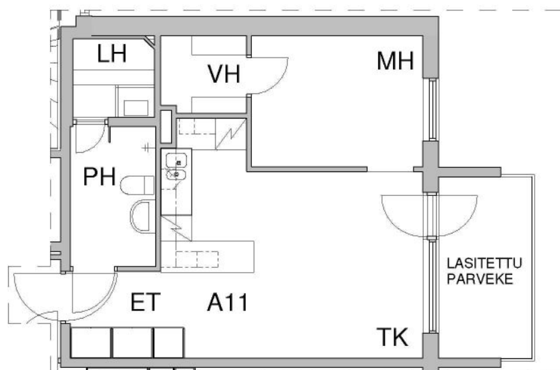
Pohjapiirros, 1:100
