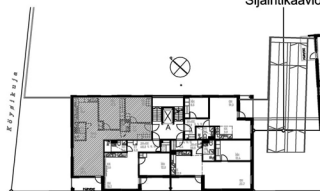
Sijaintikaavio
