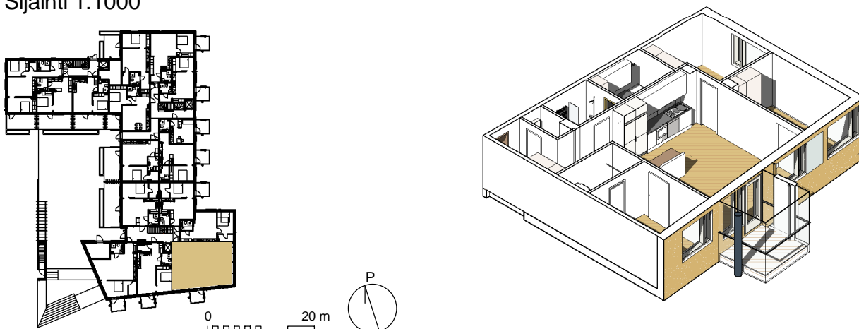
Sijainti 1:1000
