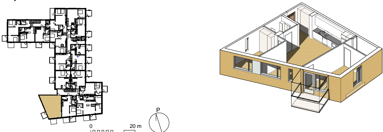
Sijainti 1:1000
