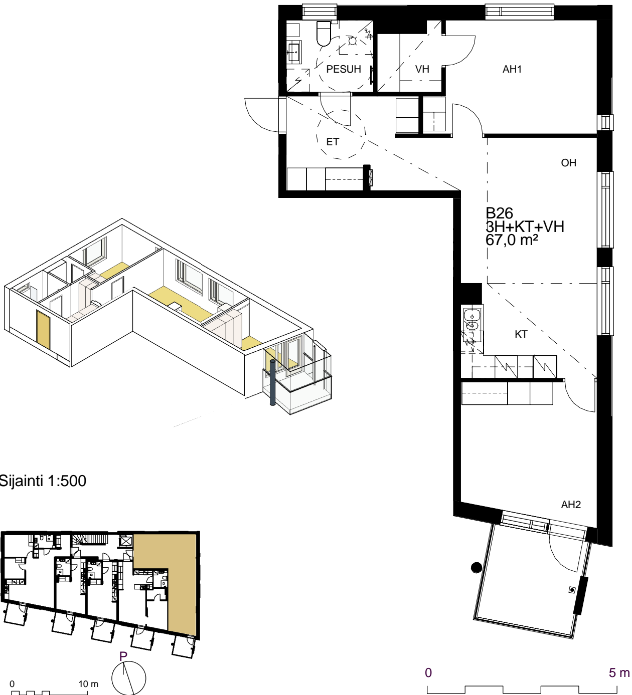
Pohjapiirros 1:100
