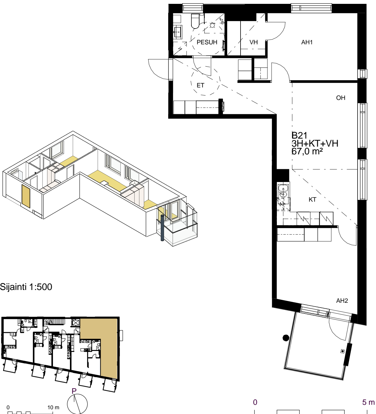
Pohjapiirros 1:100
